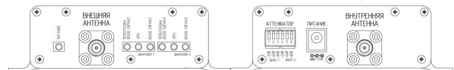
Панель индикации
