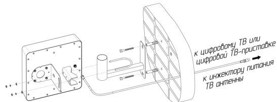
Рисунок 2 – Монтаж антенны на стеновом кронштейне
