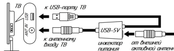
Схема 2 – Подключение активной телевизионной антенны через USB-инжектор питания
