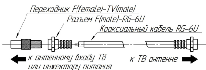
Схема 1 – Сборка антенного кабеля
