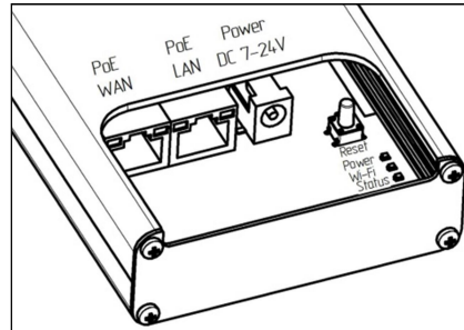
Схема 5 – Расположение портов и индикаторов роутера
