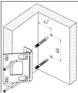
Схема 4 – Монтаж кронштейна
