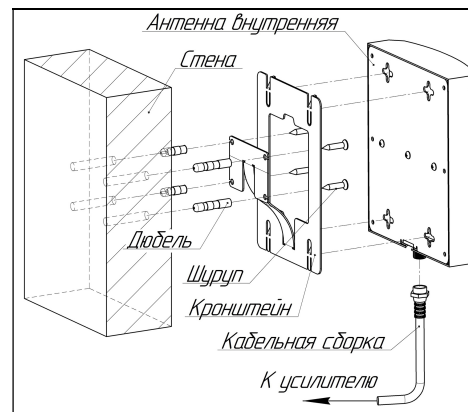
Схема 2 – Монтаж внутренней антенны
