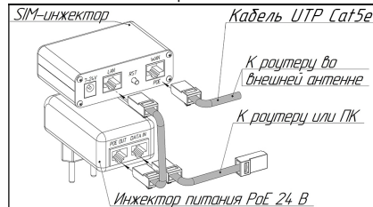
Схема 2 – PoE подключение SIM-инжектора
